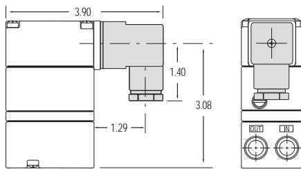
DIN 43650 Connector
